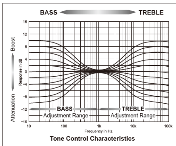
Charakterystyka regulacji tonów
